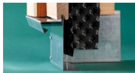
Fundamentrahmen für eine stabile Befestigung
