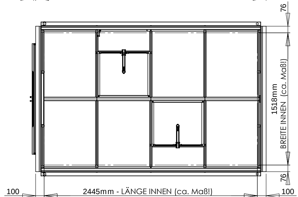
ZEICHNUNG REGATTA 264 cm
