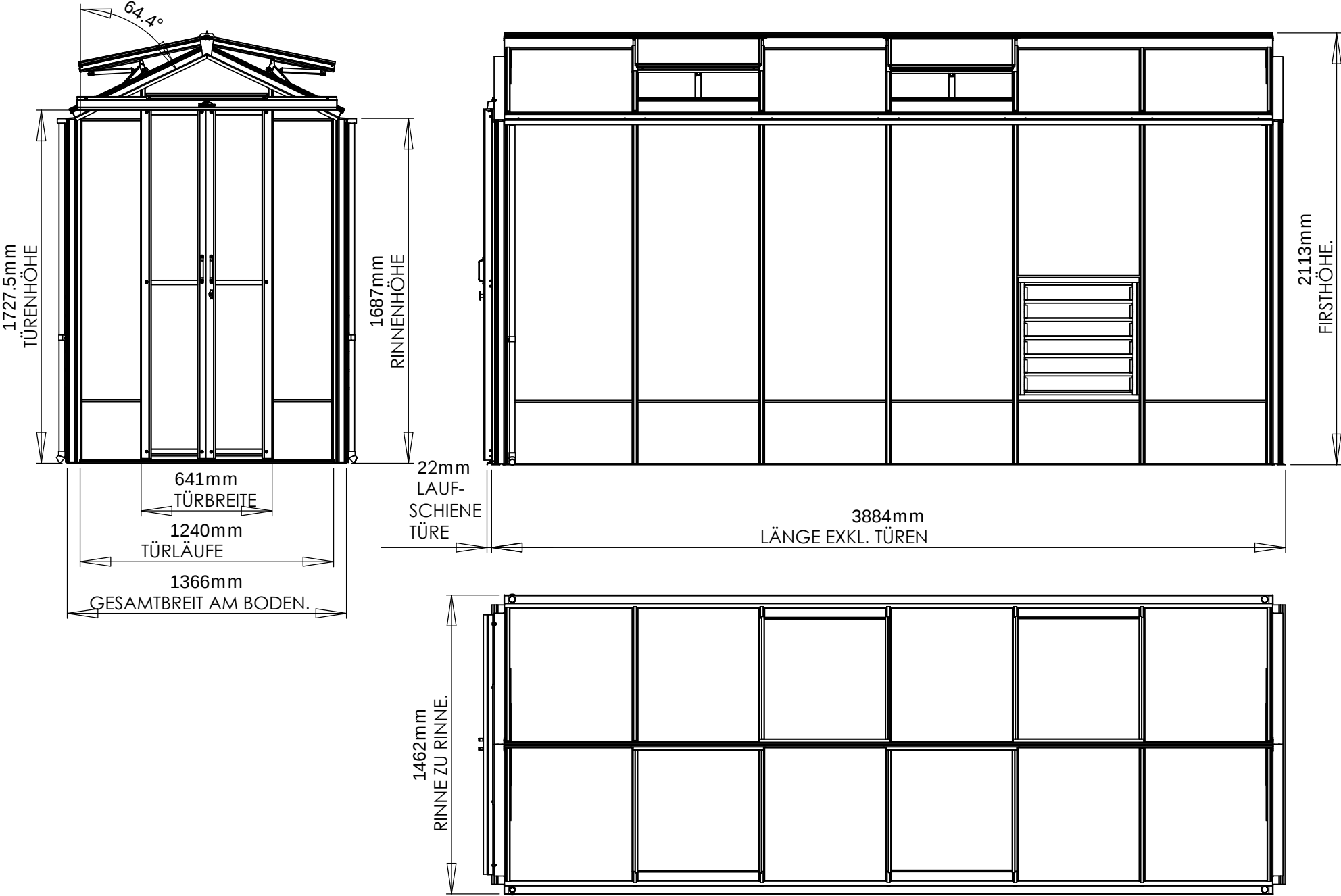
ZEICHNUNG ROWTON 387 cm
