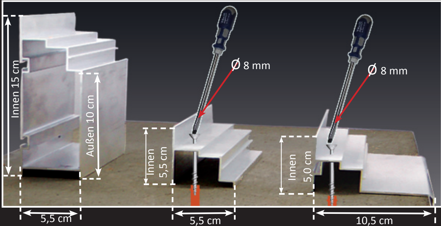
Alu-Bodenprofil
